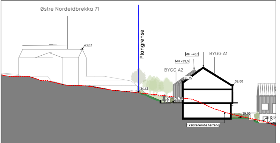
Snitt E
