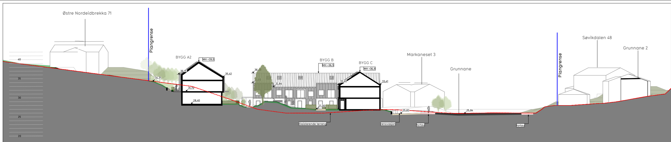
Snitt C
