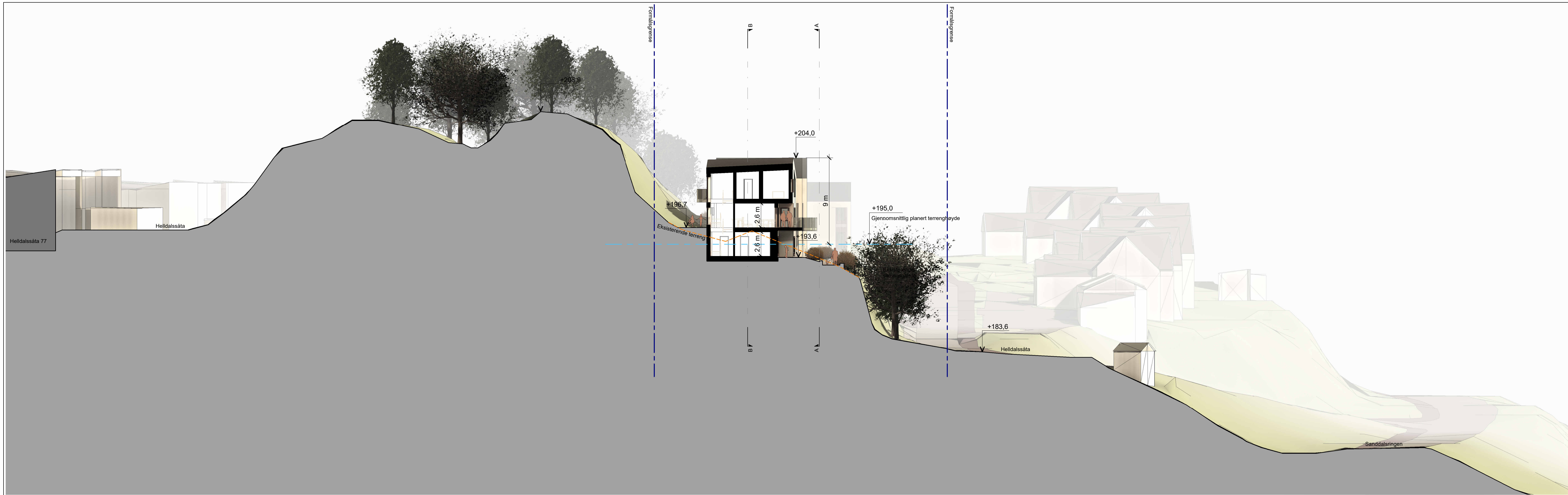
Snitt I-I 1 : 200
