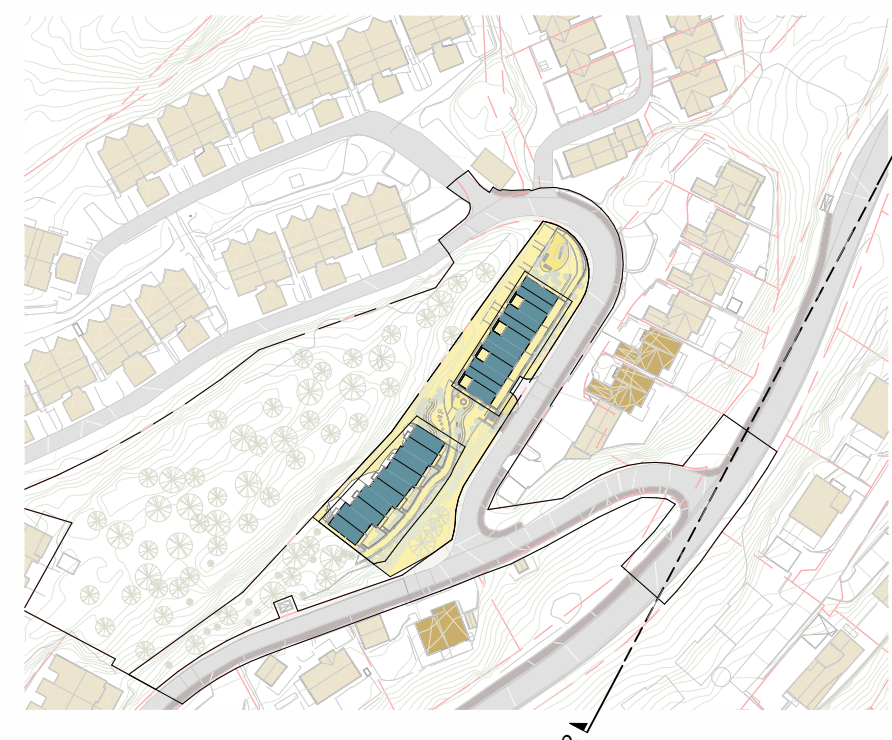
Lokaliseringsfigur - Oppriss 2 1 : 2000
