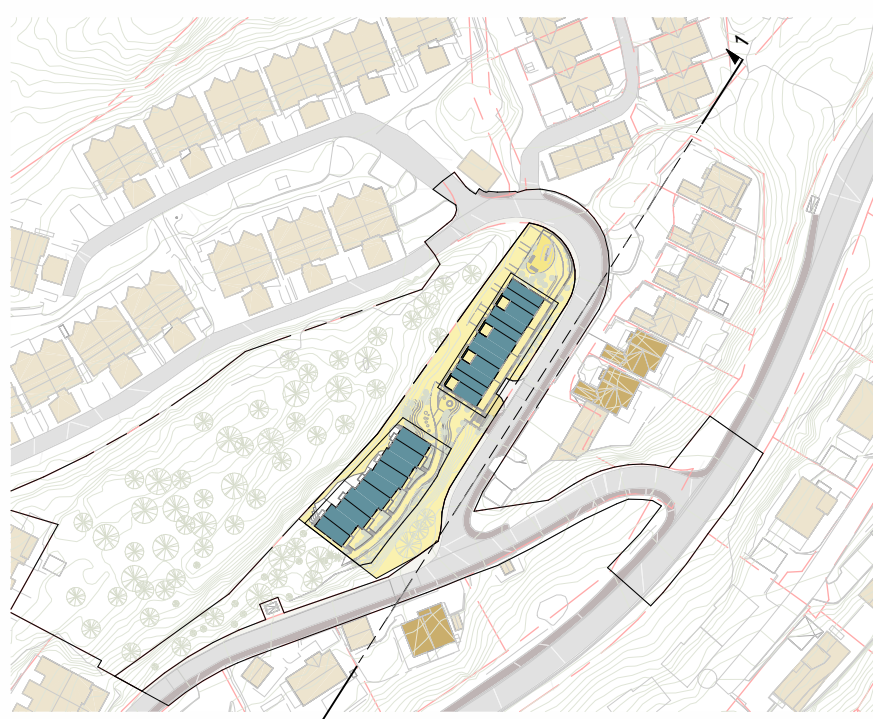
Lokaliseringsfigur - Oppriss 1 1 : 2000
