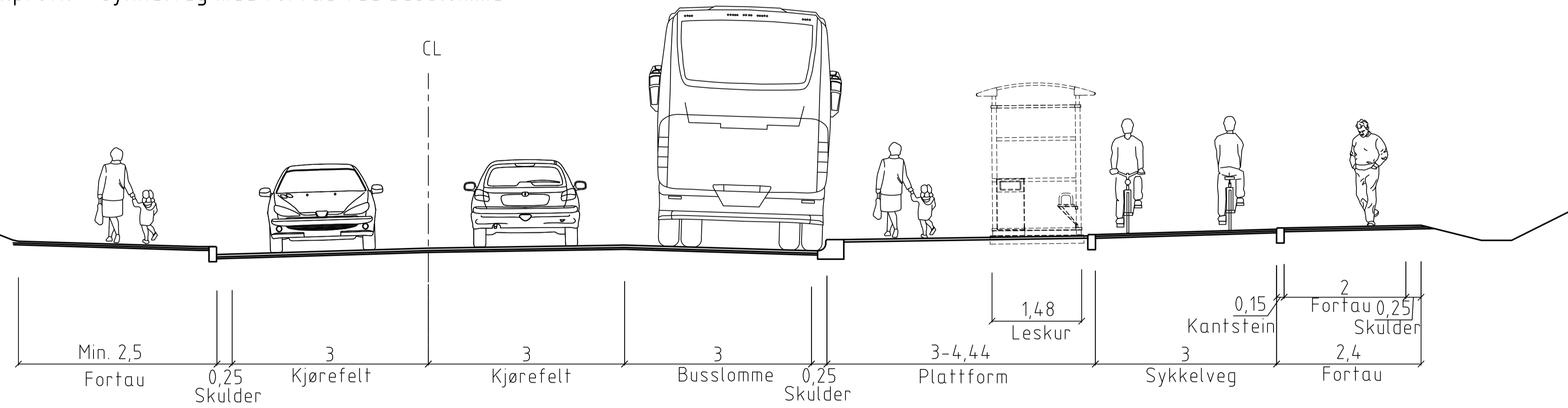
Normalprofil - sykkelveg med fortau ved busslomme
