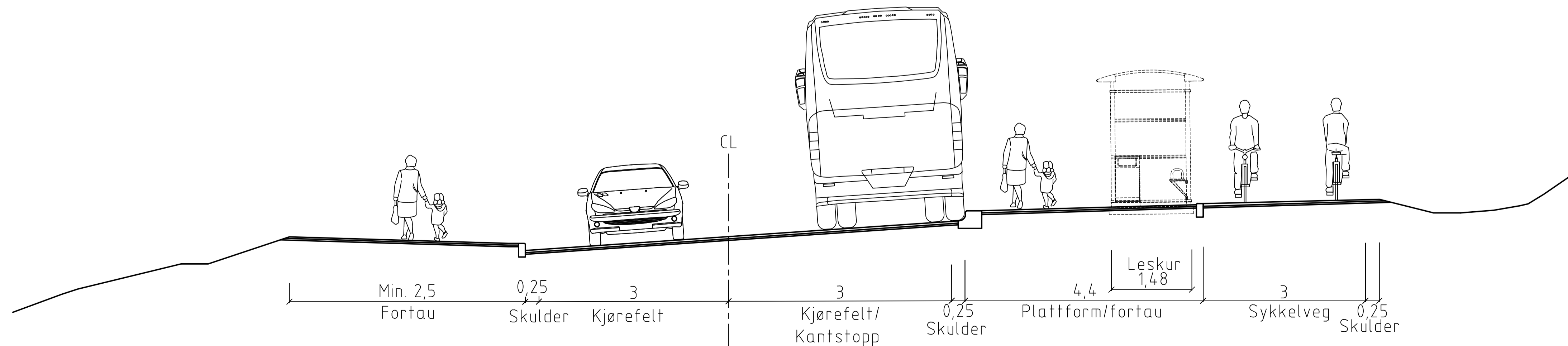
Normalprofil - sykkelveg med fortau ved kantstopp for buss
