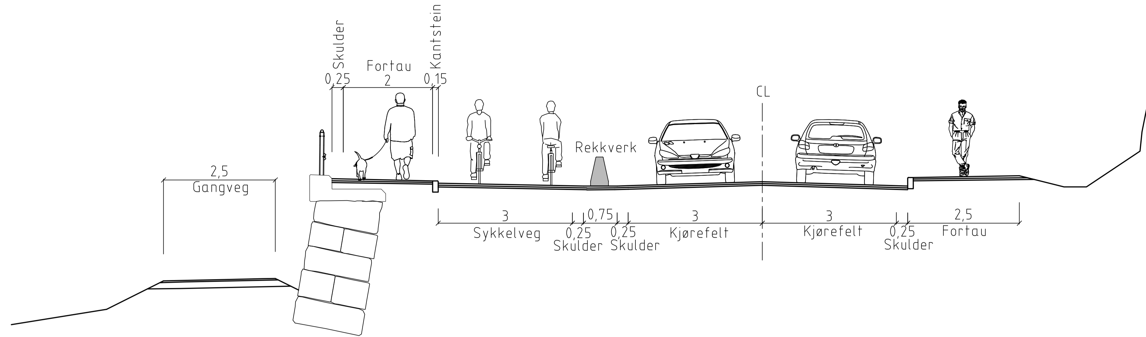
Normalprofil - sykkelveg med fortau ved mur
