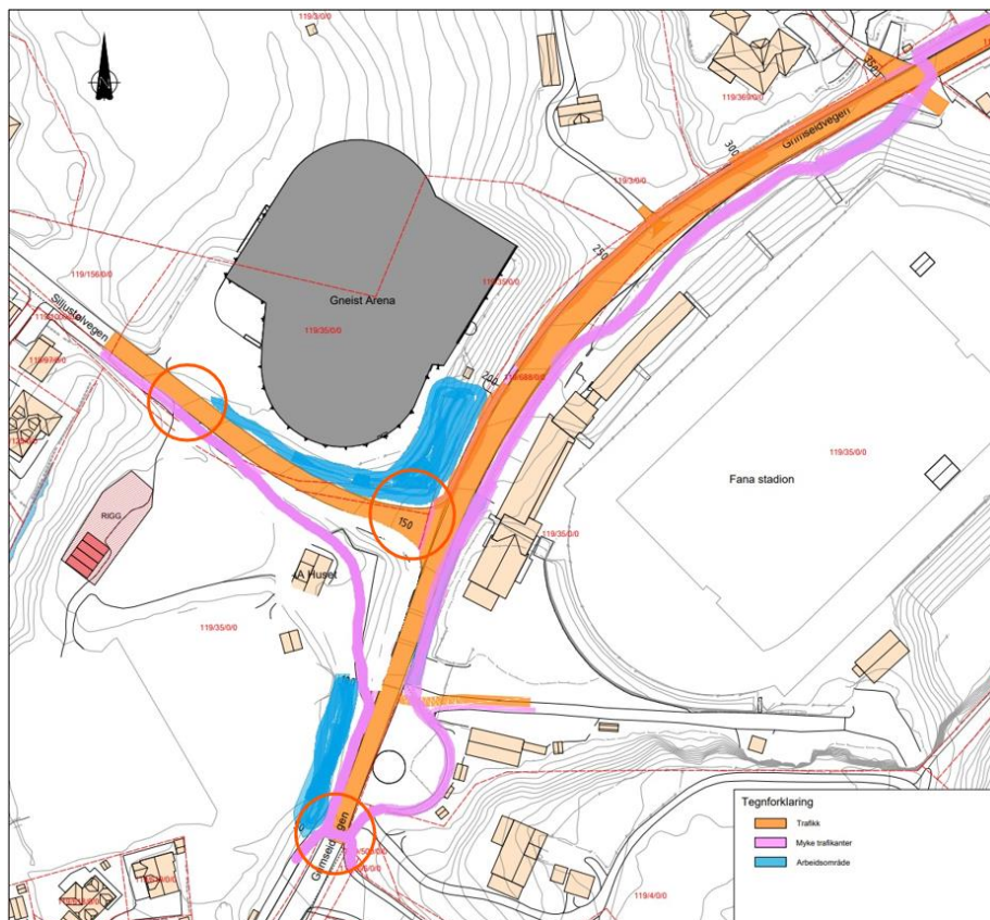
Figur 3 - skisse midlertidige gangveier og områder med manuell trafikkdirigering
