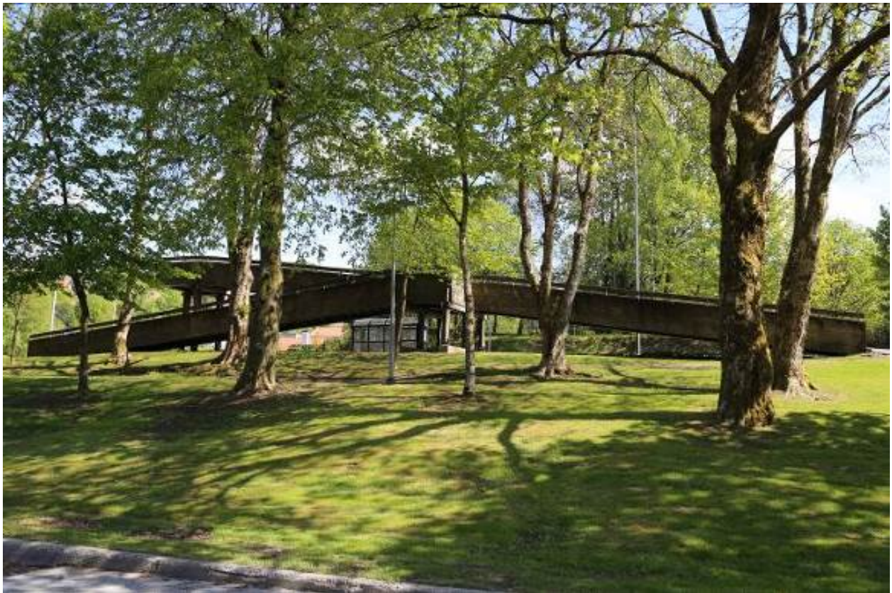
Gangbroen over Storetveitvegen i limtre.
