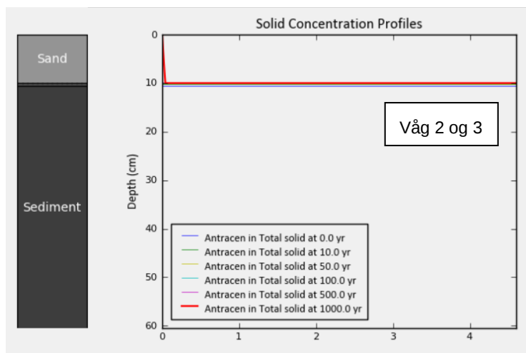
Figur 33 Resultater fra modelleringen av det kjemiske isolasjonslag med en kombinasjon av 10 cm sand og 0,5 cm (2 kg/m 2 ) aktivt kull for antracen for delområde Våg 2/Våg 3. X-aksen er kun vist opp til øvre grense for tilstandsklasse II (4,6 µg/kg for antracen). Kravet overholdes dersom rød linje (1000 år) krysser y-aksen under 5 cm dybde. Modelleringen viste de samme resultatene for de andre delområdene.
