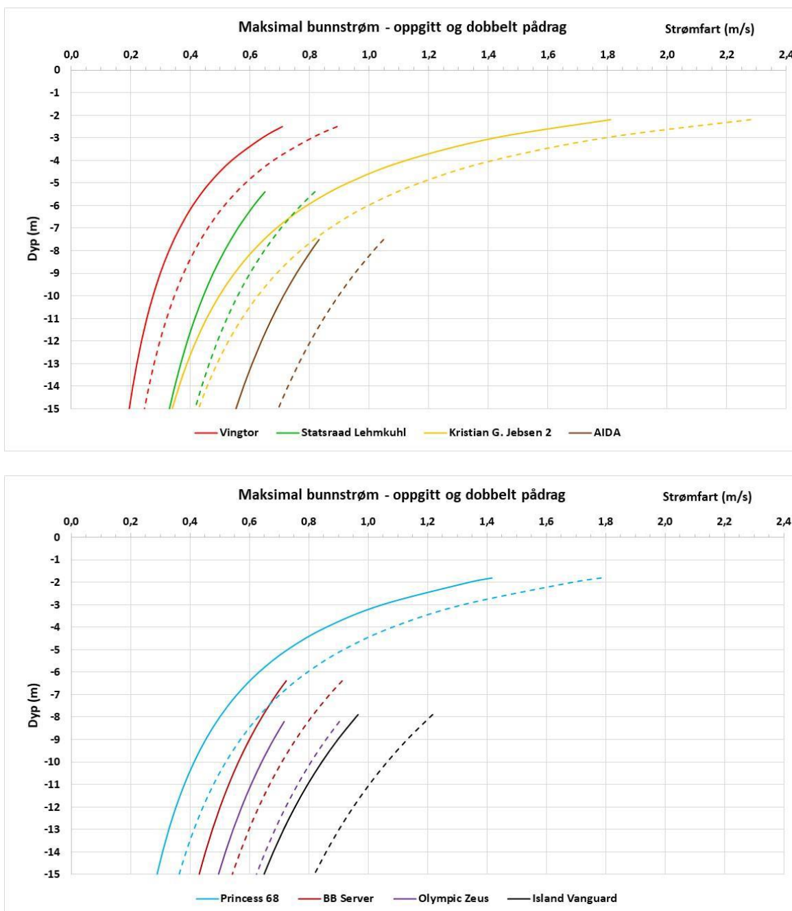
Figur 35 Maksimal propellstrøm ved bunnen for oppgitt motorpådrag (heltrukken kurve) og dobbelt motorpådrag (stiplet kurve) for vandyp ned til 15 m (Eidnes, 2021).
