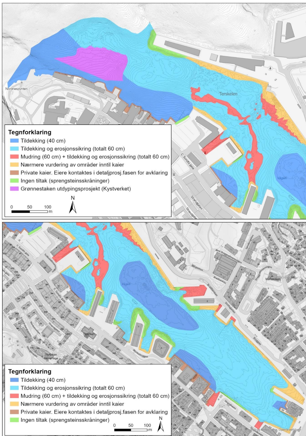
Figur 37 Foreslått tiltaksløsning for Vågen. Dybdekoter med 0,5 m ekvidistanse er vist. Det henvises til Figur 7 for oversikt over kainavn rundt Vågen.
