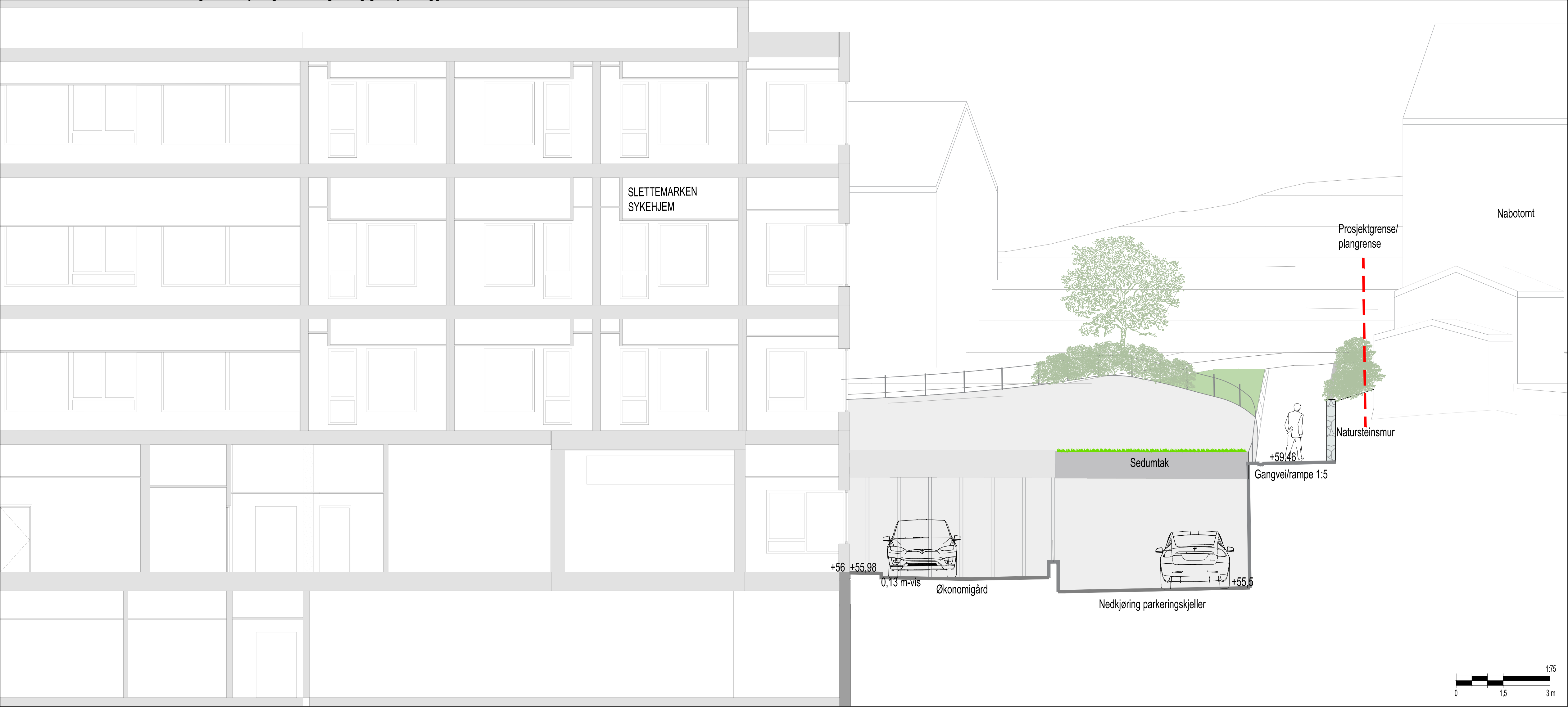
PRINSIPPSNITT H-H' - Tversnitt - Gangvei/Nedkjøring Økonomigård og garasjeanlegg
