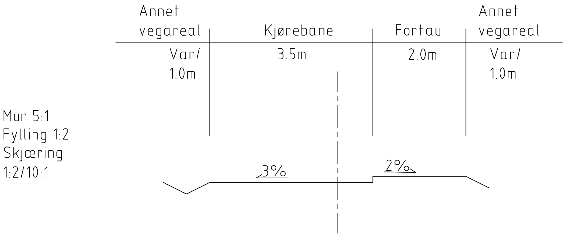
Typisk normalprofil Hegrenesveien (68300) Ensidig fortau
