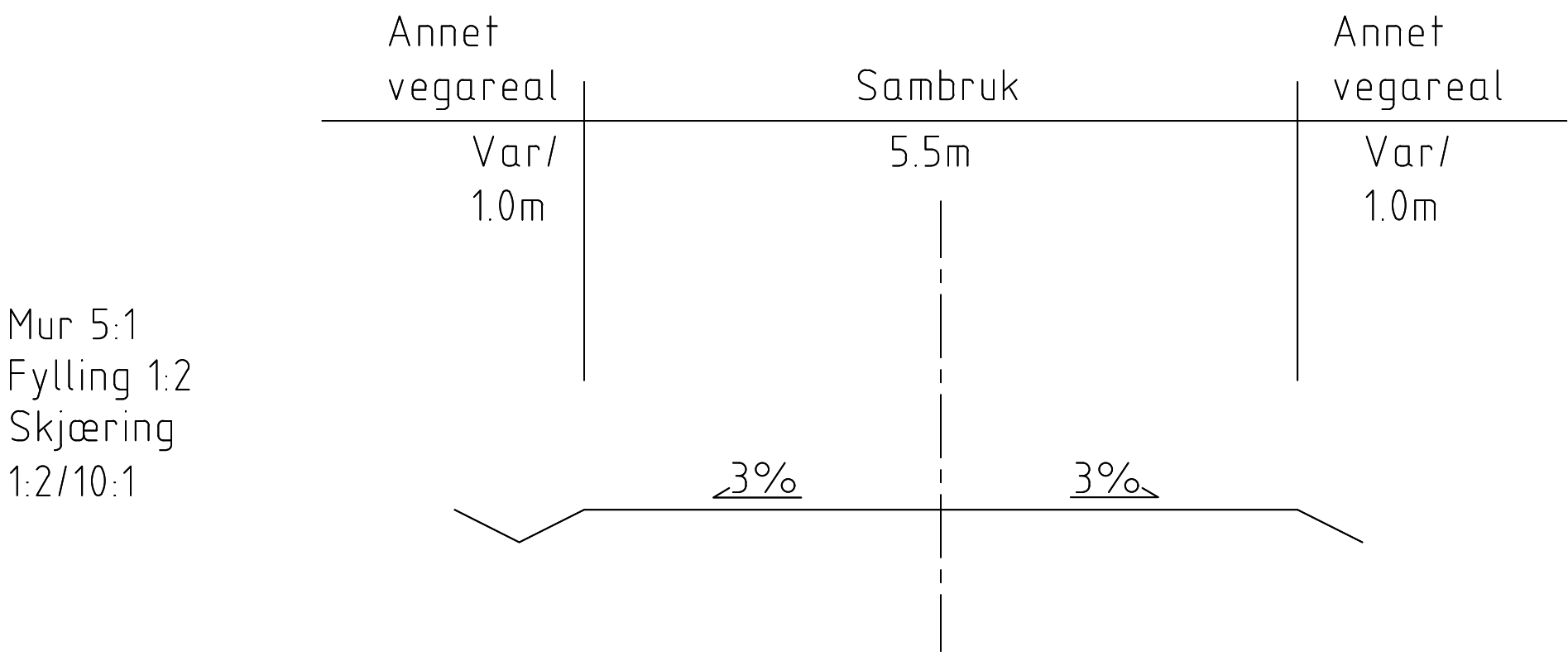
Typisk normalprofil Hegrenesveien (68300) Sambruksgate
