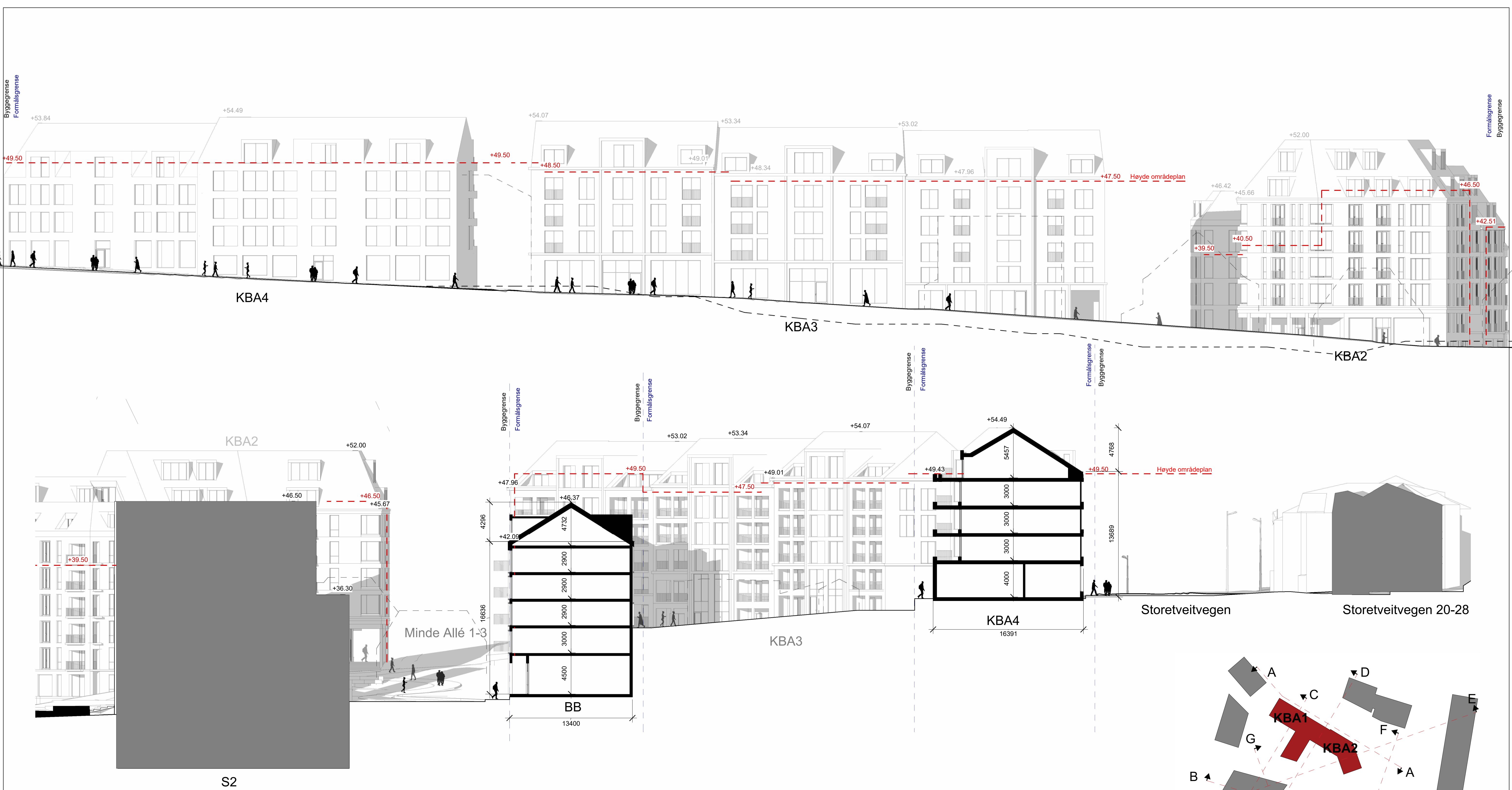
2 Høydesnitt G 1 : 200
