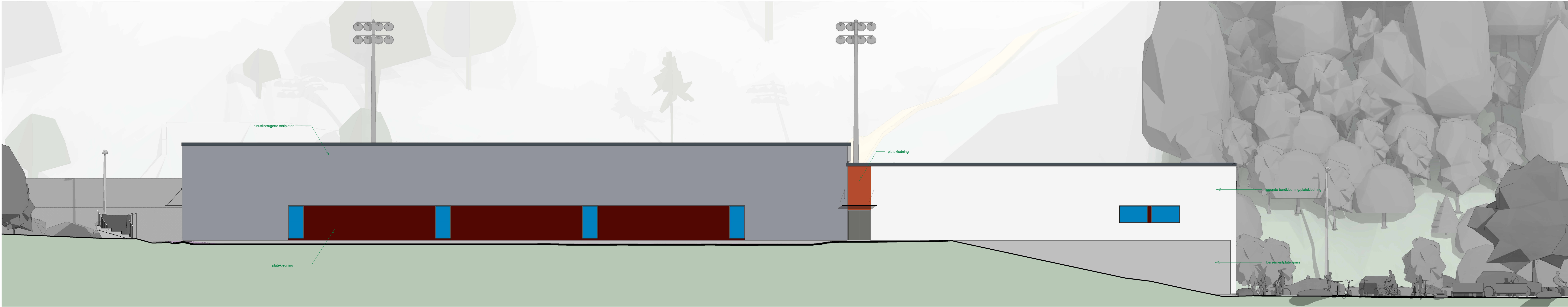
1 Fasade mot vest 1 : 100
