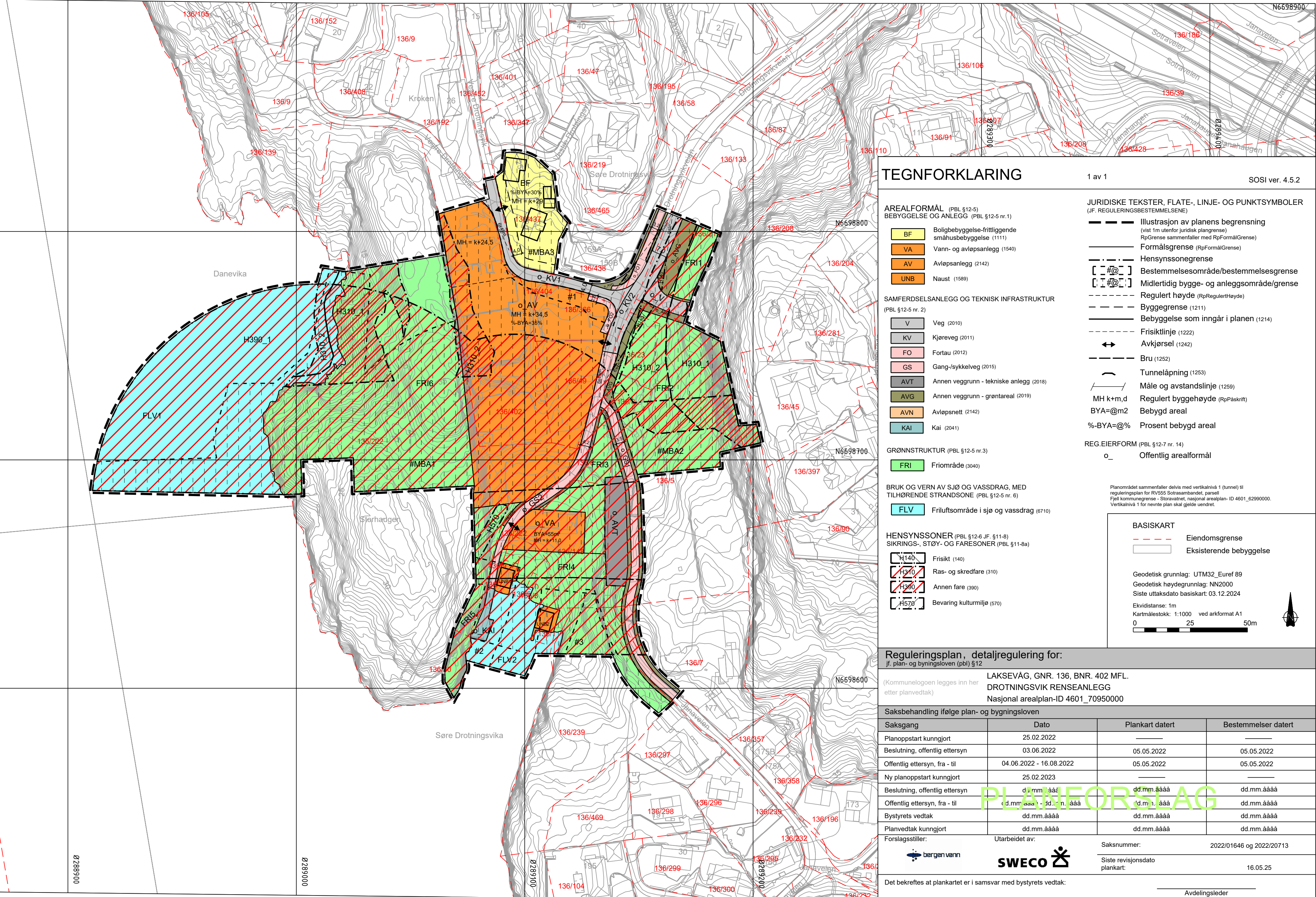
Regulering på grunnen, vertikalnivå 2 Målestokk 1:1000
