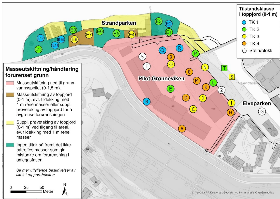
Figur 64 Oversikt over masseutskiftning/massehåndtering av forurenset grunn i Pilot Grønneviken og Strandparkens tiltaksområde. Tiltaksbeskrivelsen i figuren er ikke komplett, og det henvises til rapport-teksten for utfyllende beskrivelse.
