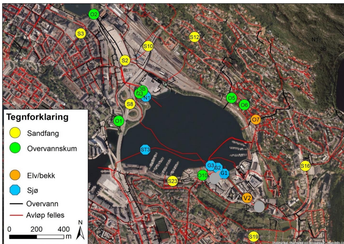
Figur 27 Oversikt over vannprøvelokaliteter (fra COWI, 2019)
