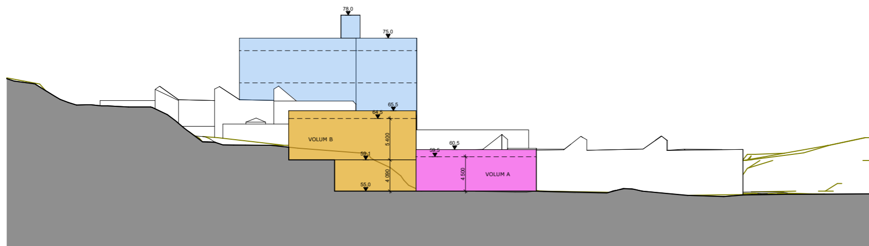
Snitt B 1:500
