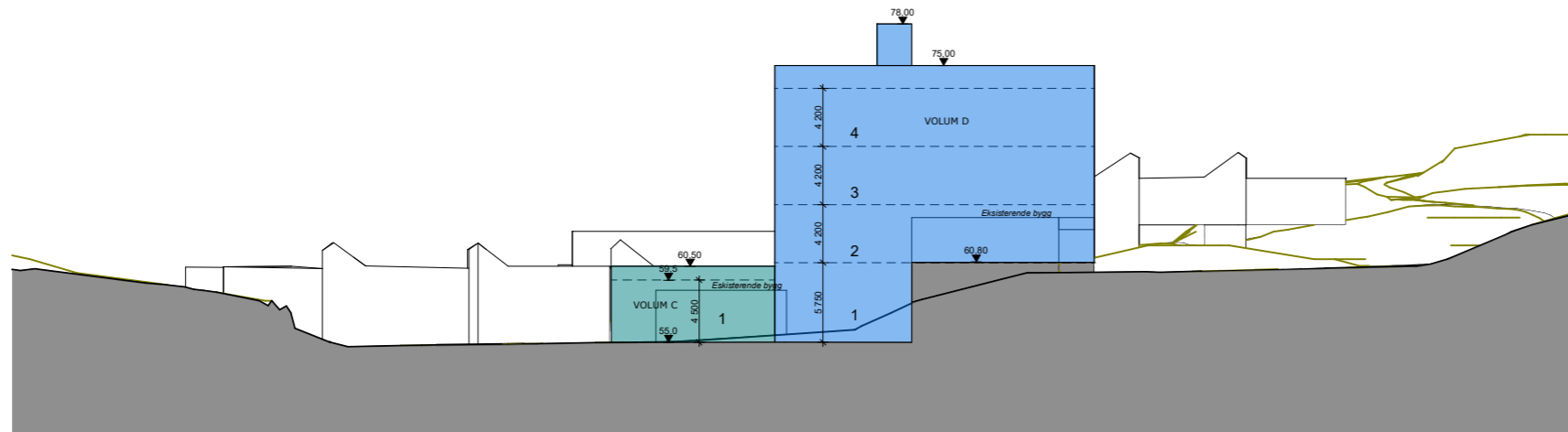
Snitt A 1:500
