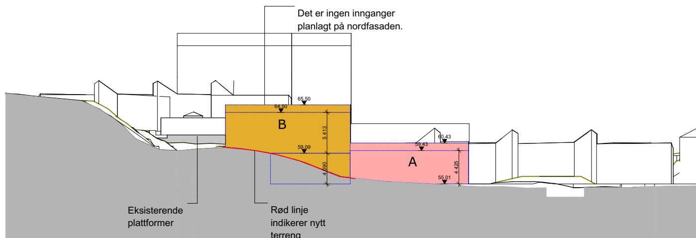
Snitt C - Alternativ justering av reguleringsforslag 1:500
