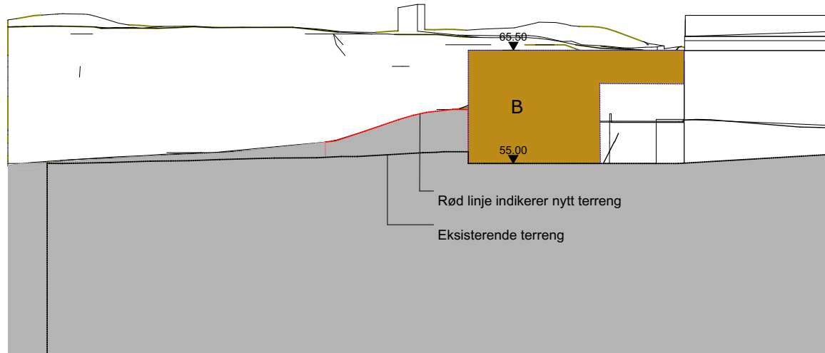
Snitt D - Alternativ justering av reguleringsforslag 1:500
