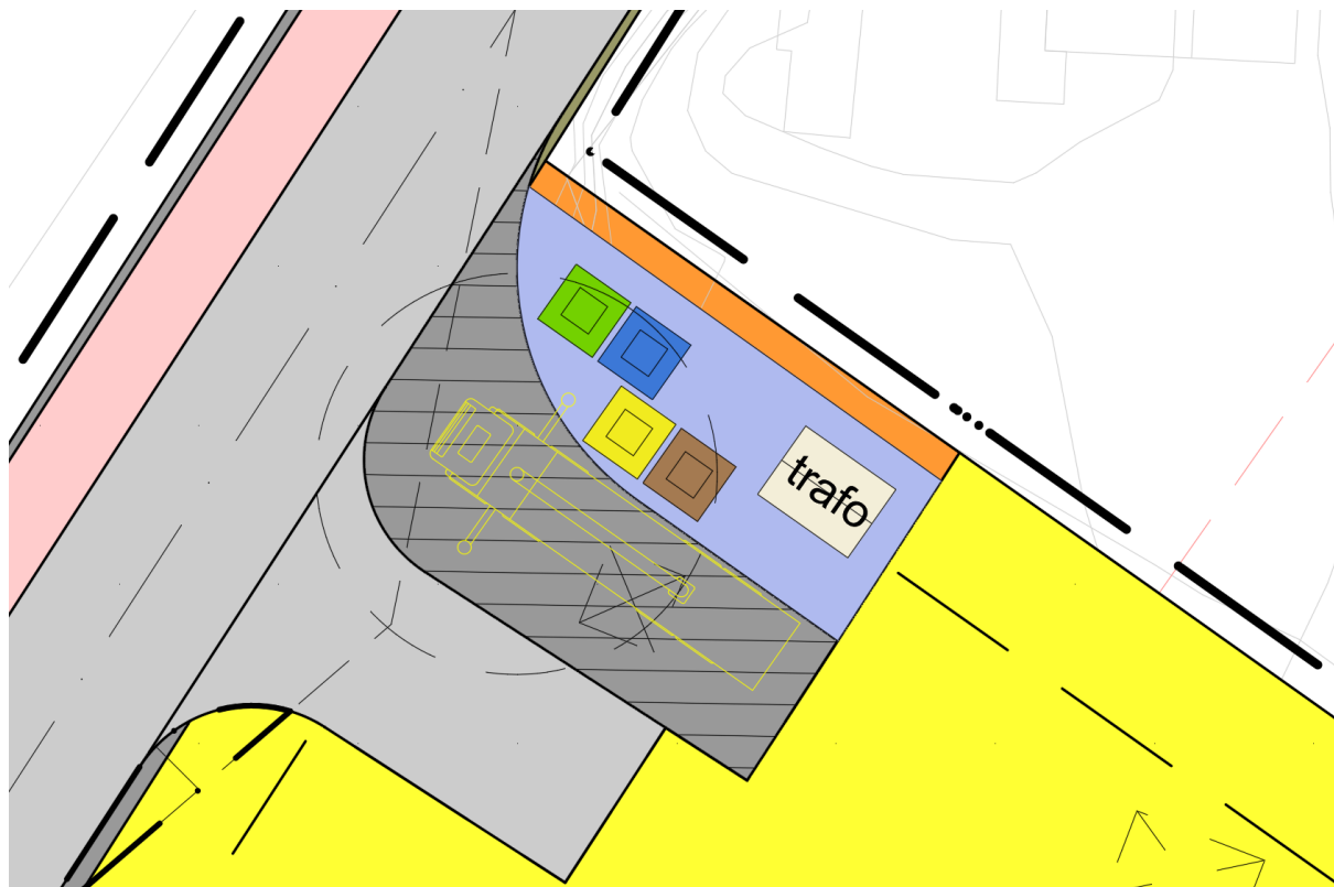
Figur 17: Skisse av hvordan renovasjonsbil kan stille seg opp ved tømming. Skravur viser oppstillingsplass.
