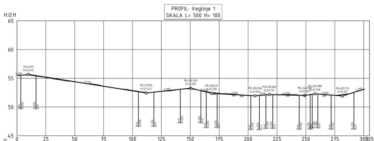
Figur 10: Lengdeprofil for tilkomst fra vest over Hjortevegen og Dyrhaugen, utkjøring nordover over Dyrhaugen.
