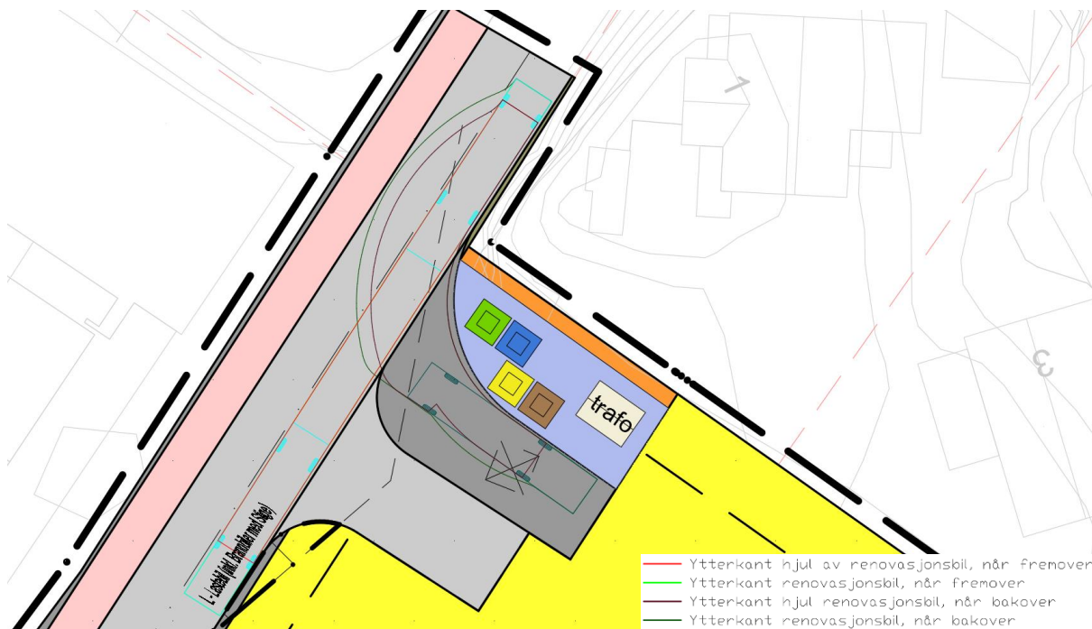
Figur 13: Tilkomst sørfra over kv.4577 Hjortevegen og o_KV.
