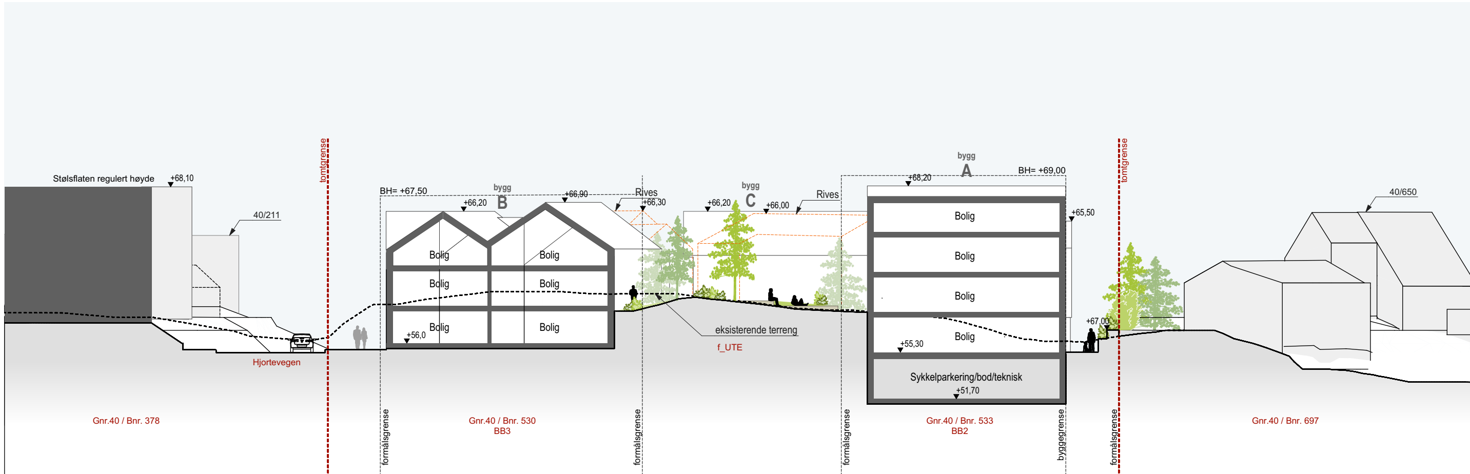
snitt BB
