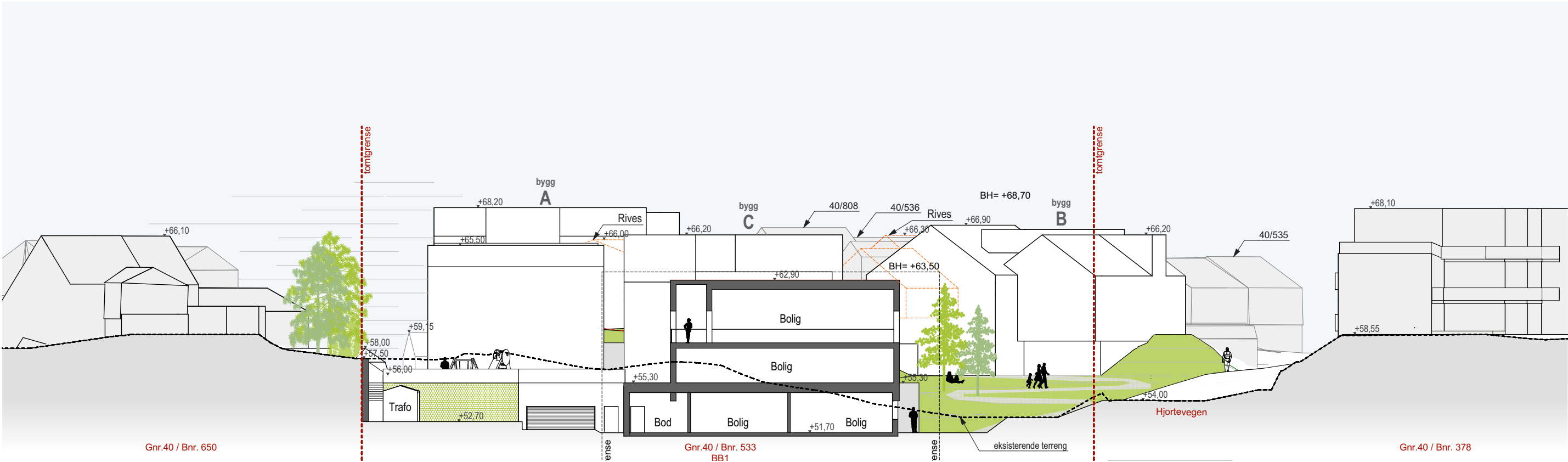
snitt CC
