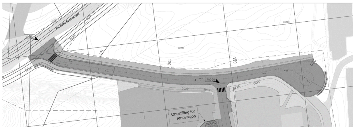
Figur 29 - Prosjektert offentlig kjøreveg Barliveien med snuhammer og avkjørsel til det nye boligområdet og parkeringsplass for Tjernet borettslag, koblet på regulert fylkesveg Spelhaugen. (Linjer fra gjeldende regulering er vist på illustrasjonen.)
