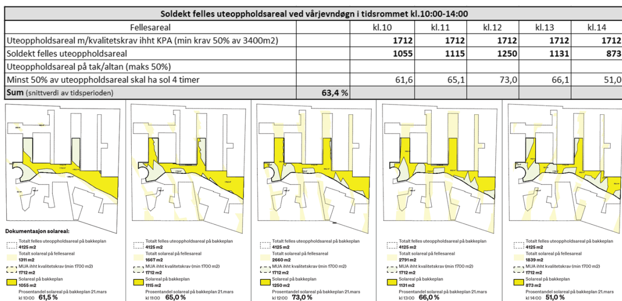
Figur 24 – Illustrasjonen viser at mer enn 50% av uteoppholdsareal på bakkeplan har sol (gult) kl. 10, 11, 12, 13 og 14.
