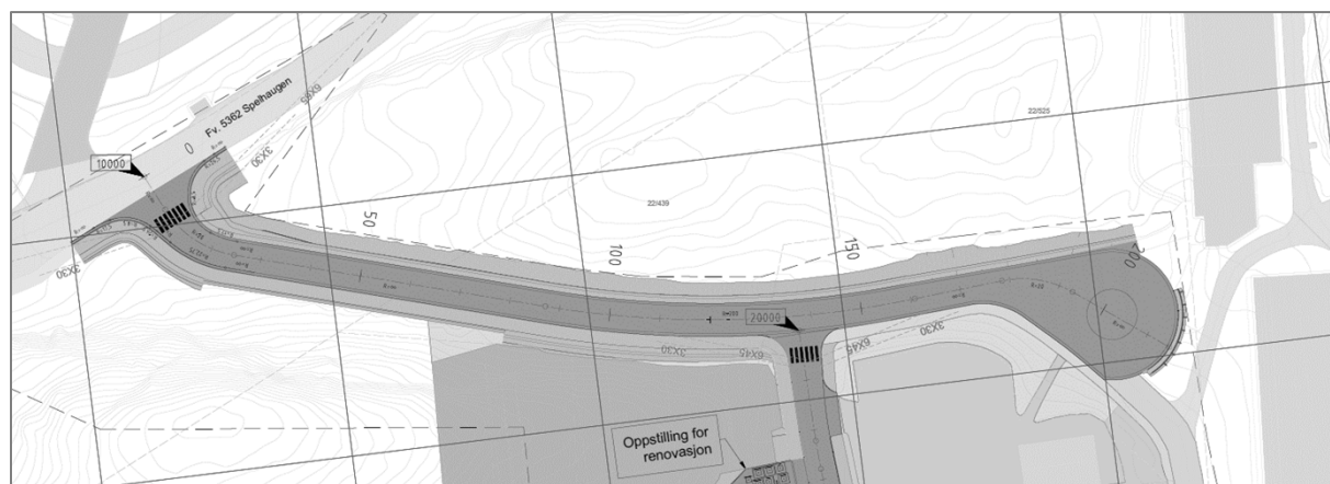
Figur 28 - Prosjektert offentlig kjøreveg Barliveien med snuhammer og avkjørsel til det nye boligområdet og parkeringsplass for Tjernet borettslag, koblet på eksisterende fylkesveg Spelhaugen.
