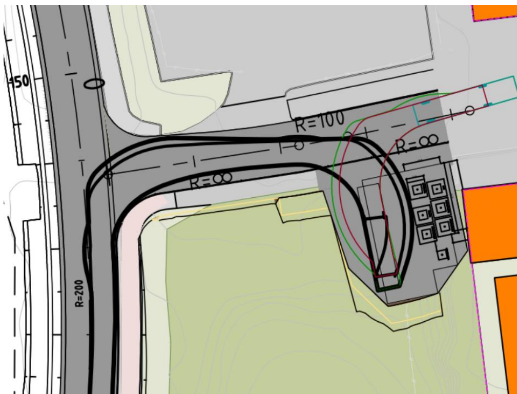
Figur 8: Sporingskurver for innkjøring til oppstillingsplass for renovasjonsbilen, med rygging mot venstre inn mot boligområde.
