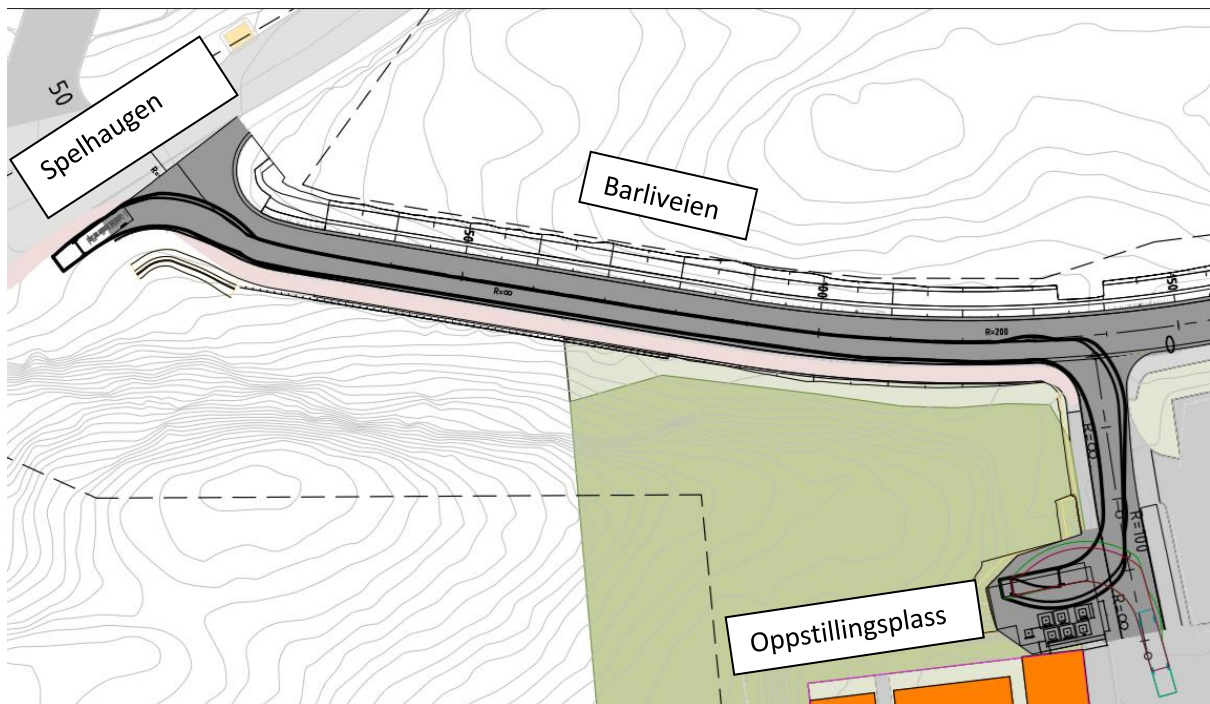
Figur 7: Sporingskurver for tilkomstvei frem til oppstillingsplass, fra Spelhaugen, via Barliveien, frem til oppstillingsplass for renovasjon
