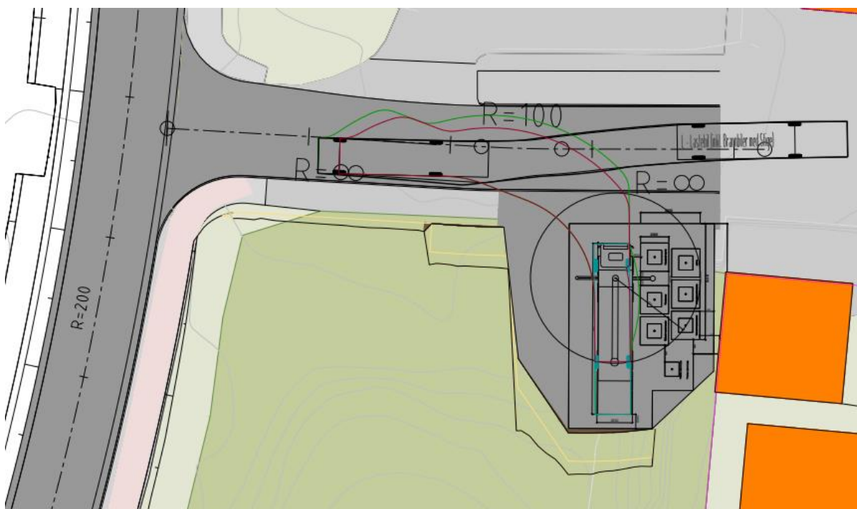
Figur 9: Sporingskurver for rygging inn på oppstillingsplass til tømmeponisjon.
