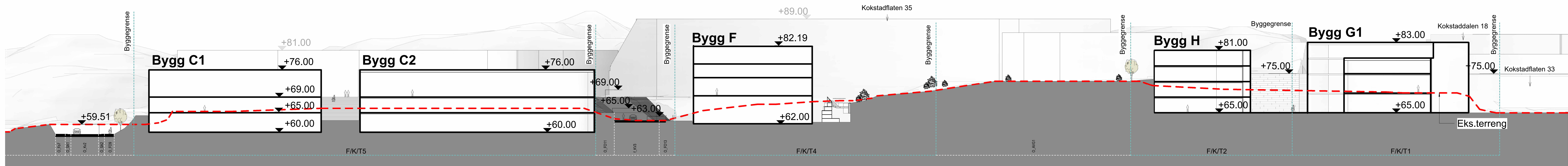
Lengdeprofil B - 1 : 350
