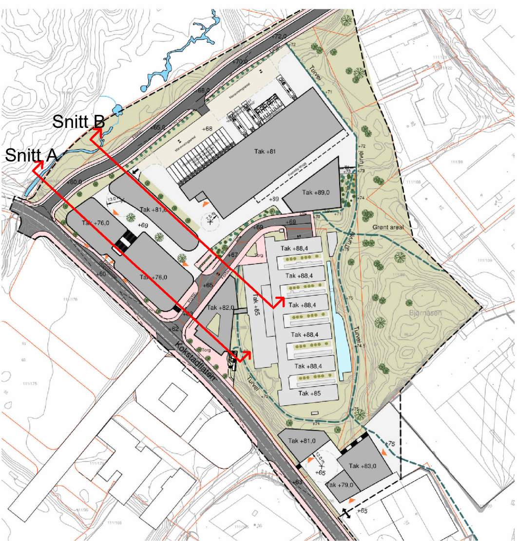
791 - Snitt oversikt 1 1 : 3000
