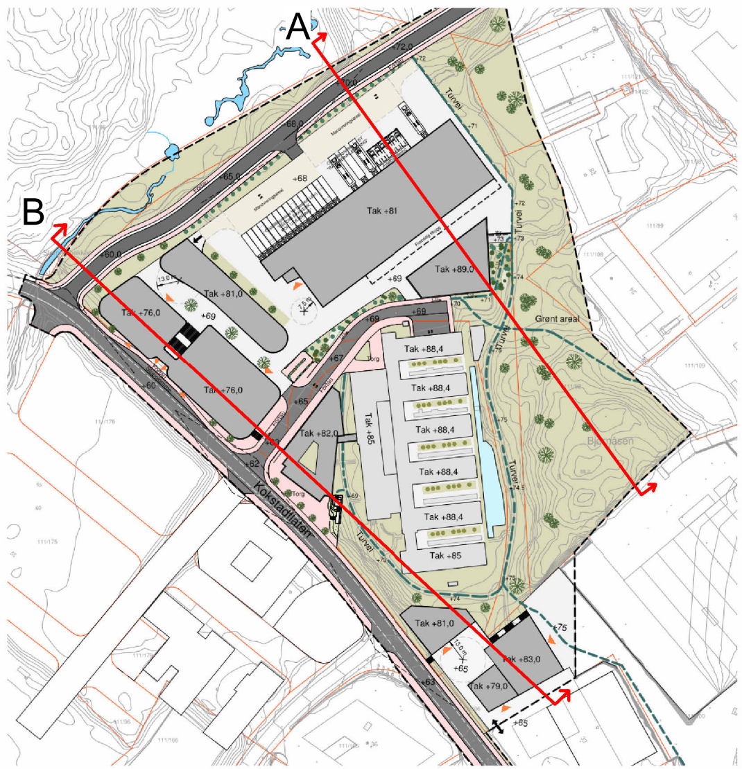
791 - Lengdeprofil 1 : 3000
