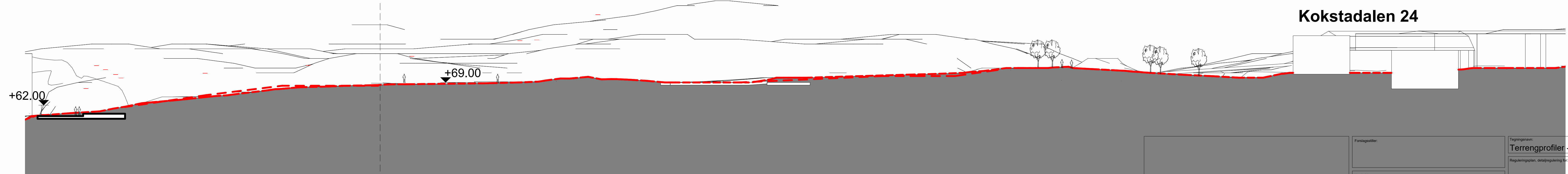
Profil D-D Eksisterende situasjon 1 : 350
