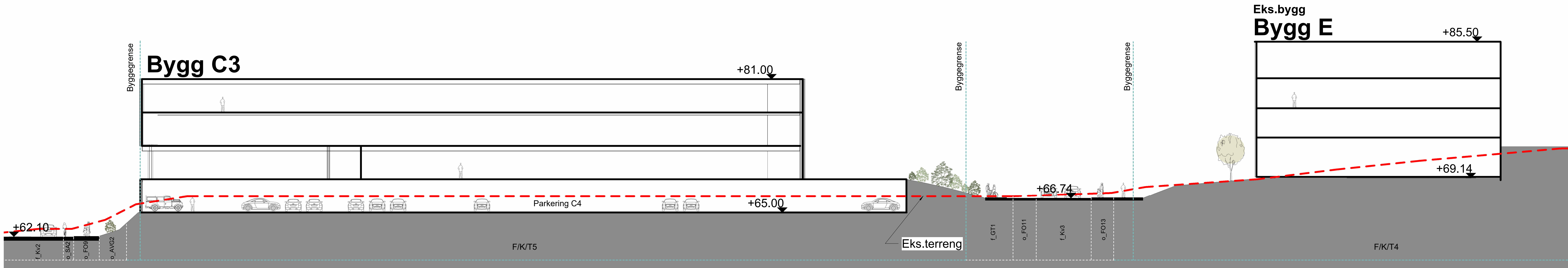
Snitt B 1 : 200
