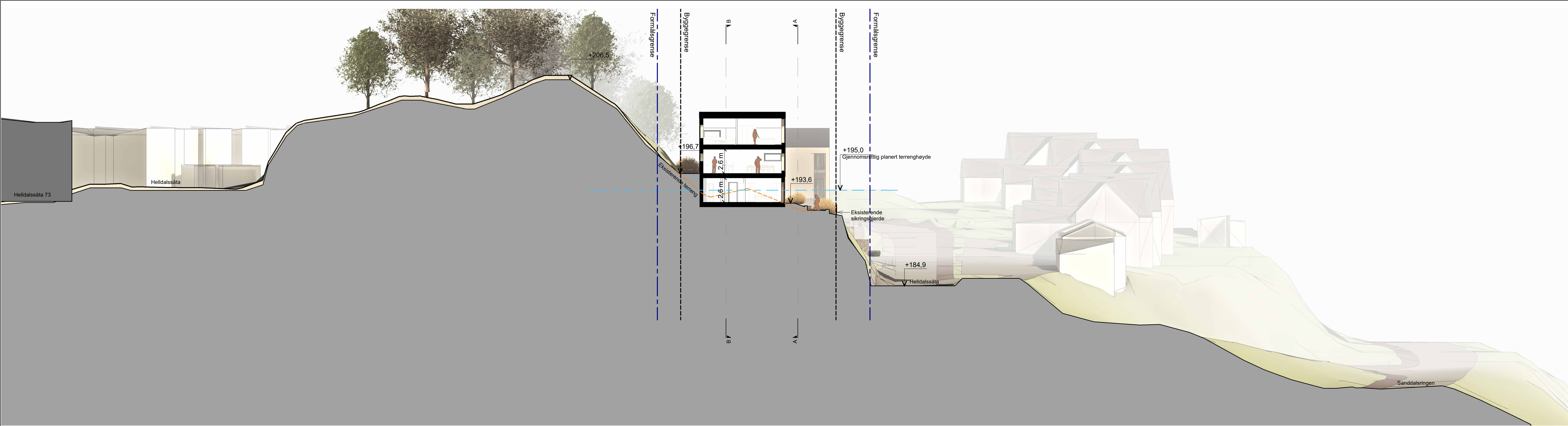
Snitt G-G 1 : 200
