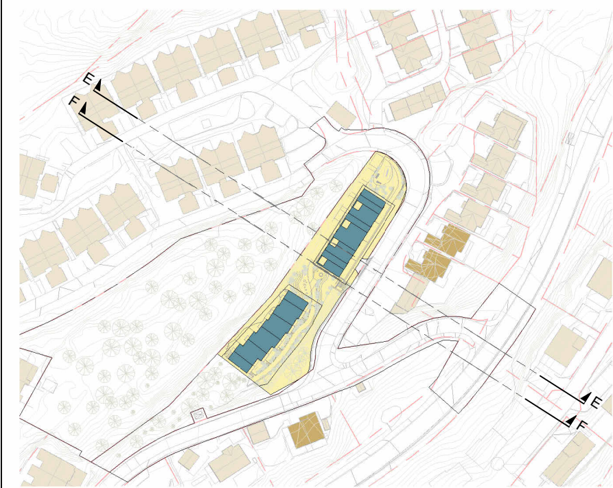
Lokaliseringsfigur - Snitt E og F 1 : 2000
