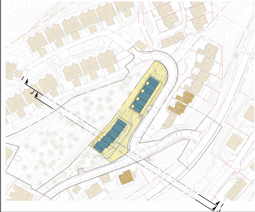
Lokaliseringsfigur - Snitt I og J 1 : 2000
