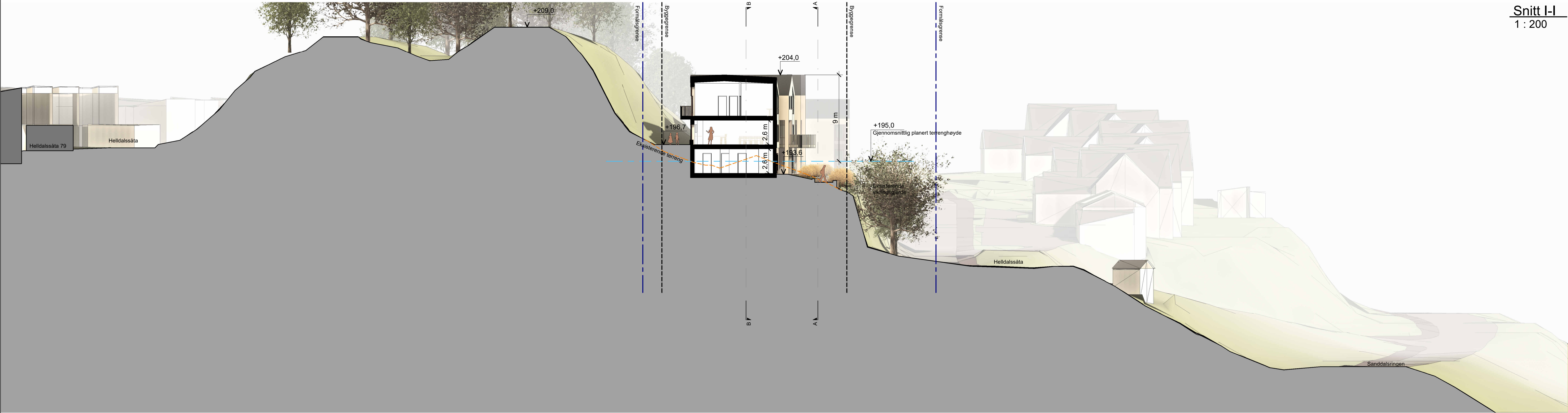
Snitt J-J 1 : 200
