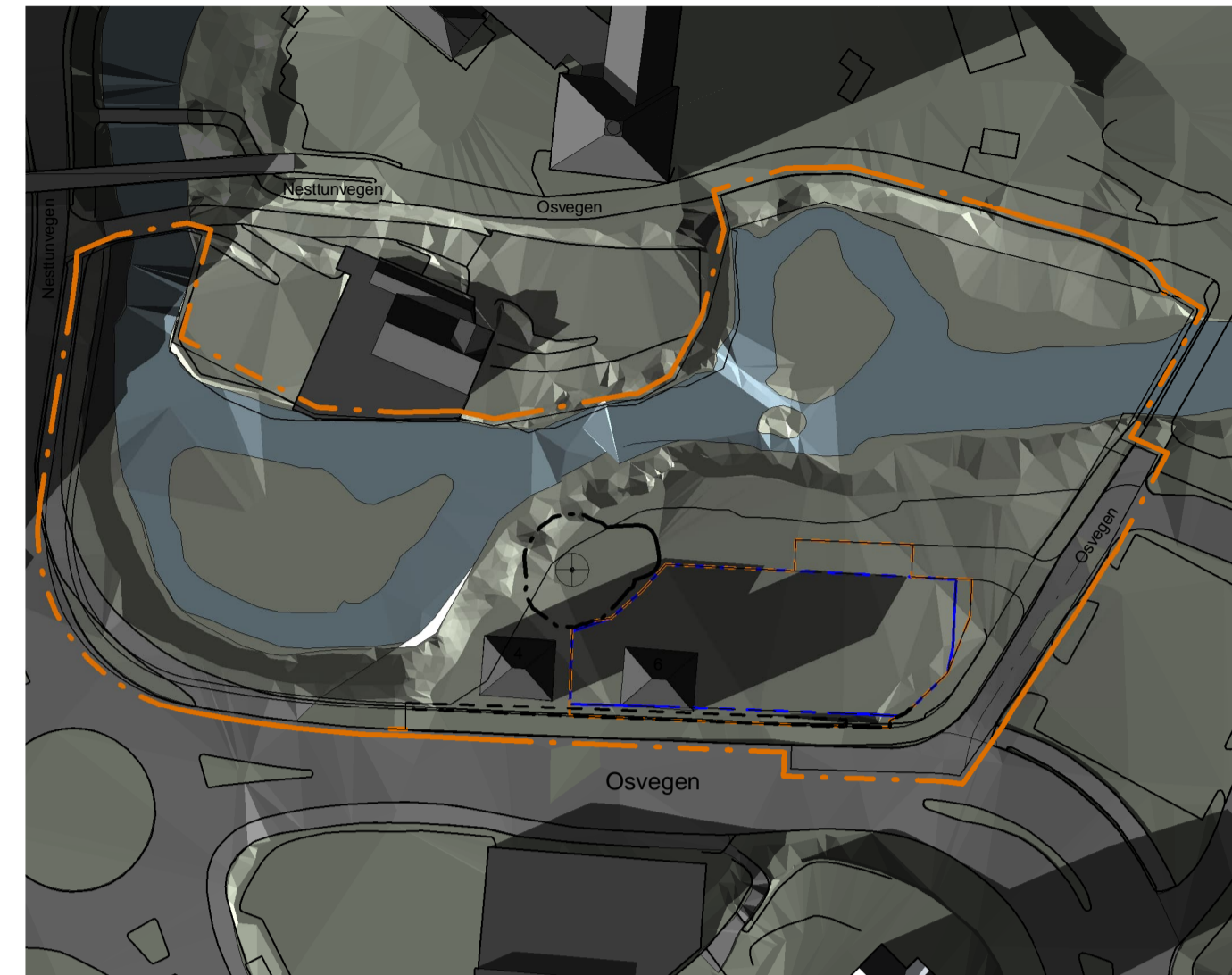
Sol/Skygge studie Vårjevdøgn k118 Idag
