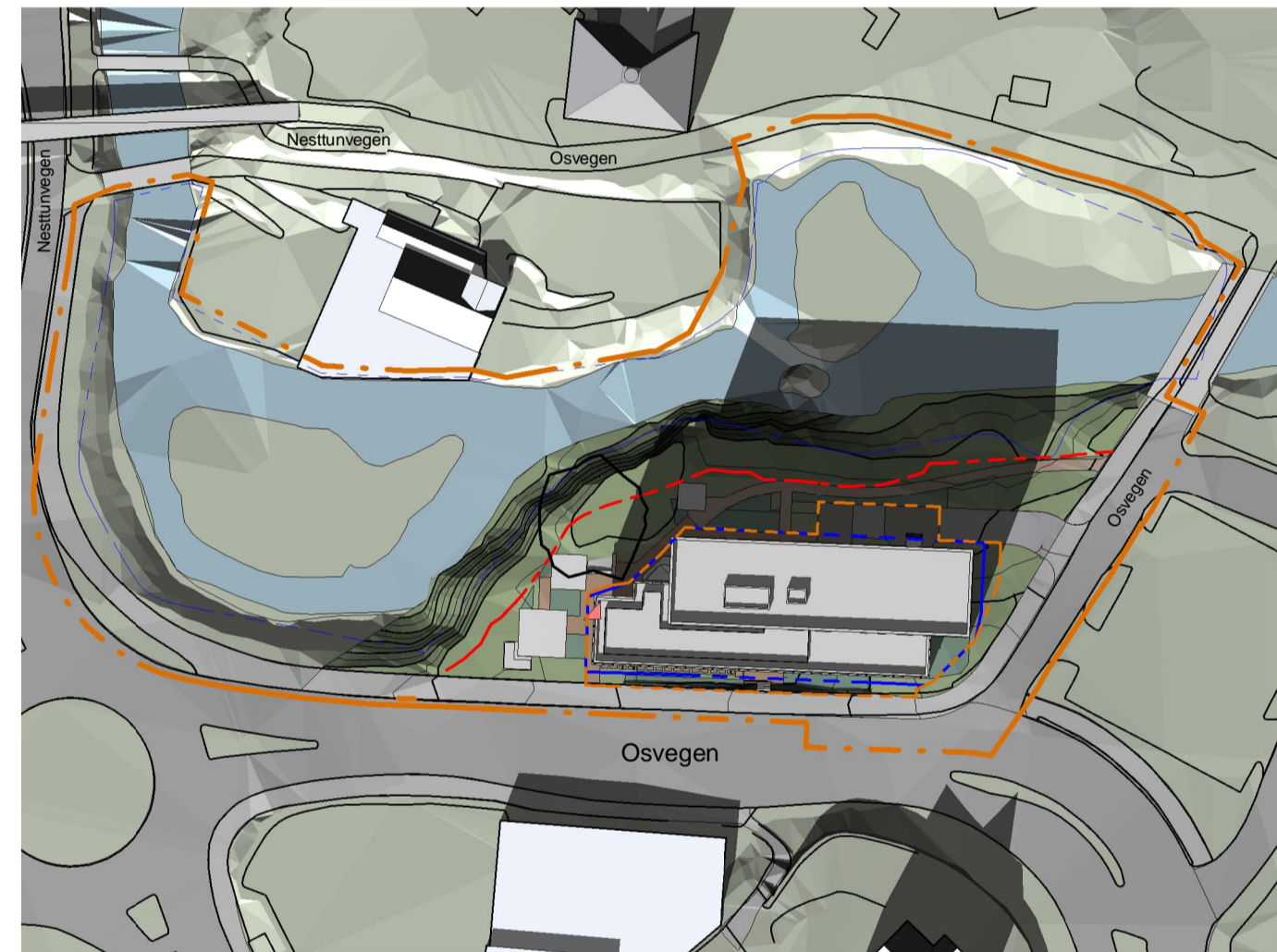
Sol/Skygge studie Vårjevdøgn k115 Etter
