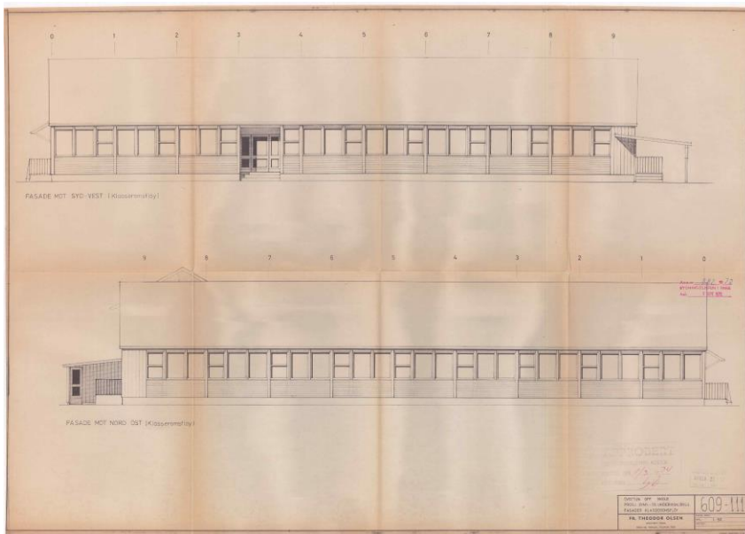
Figur 4-80 Fasader undervisningsbygget, fra byggesøknad fra 1972. Arkitekt Fr. Theodor Olsen.
