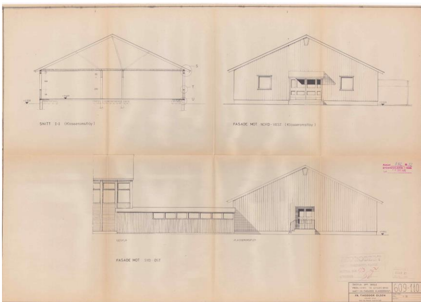
Figur 4-81 Snitt og fasader, kortvegger av undervisningsbygget, i byggesøknad fra 1972. Nederste tegning viser også leskuret mot gymsalen. Arkitekt Fr. Theodor Olsen.
