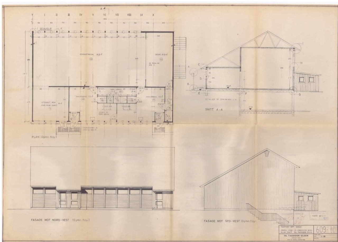
Figur 4-63 Gymsalen, plan og fasadetegninger i byggesøknad fra 1972. Arkitekt Fr. Theodor Olsen.
