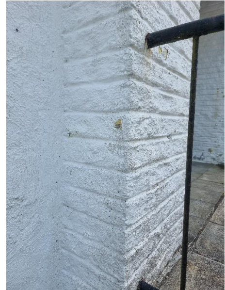
Figur 4-11 Detalj av inngangsparti. Undersøkelse viste at det var betong under pussen. Båndene er trolig ment å etterligne tegl.
