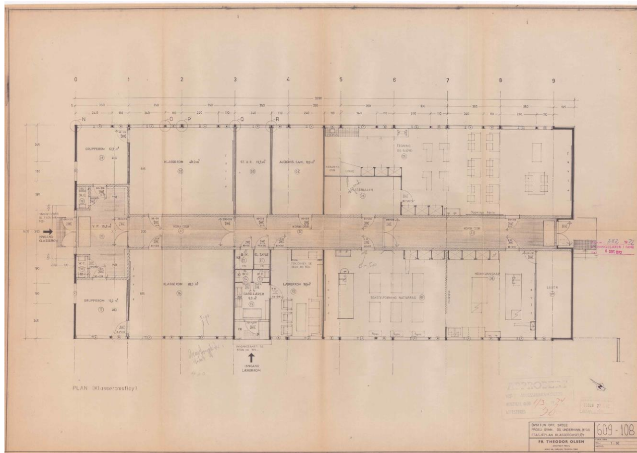
Figur 4-82 Plan over undervisningsbygget, 1972. Arkitekt Fr. Theodor Olsen.
