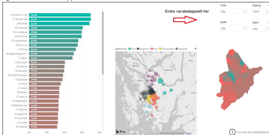
Figur 2: Endre variabeloppsett
